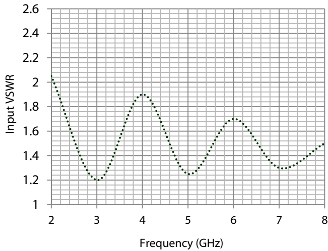
Input VSWR
