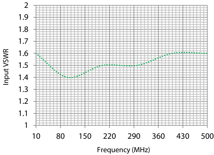
Input VSWR
