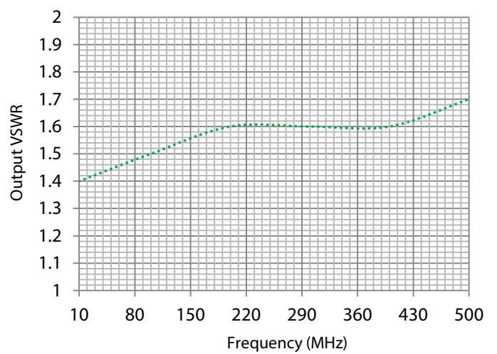
Output VSWR
