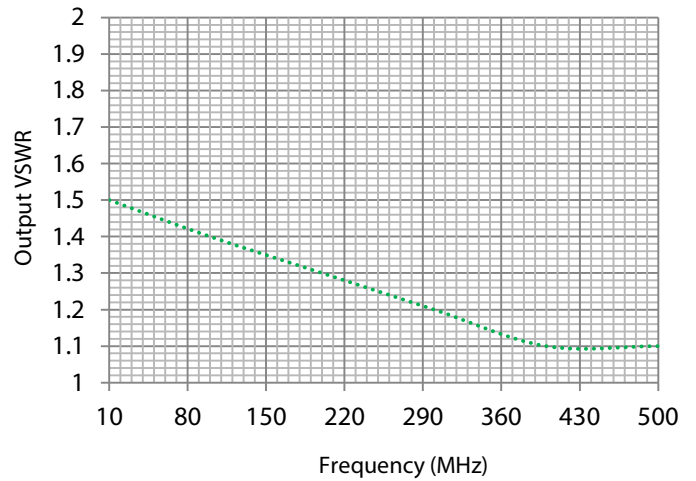
Output VSWR
