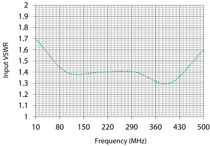
Input VSWR
